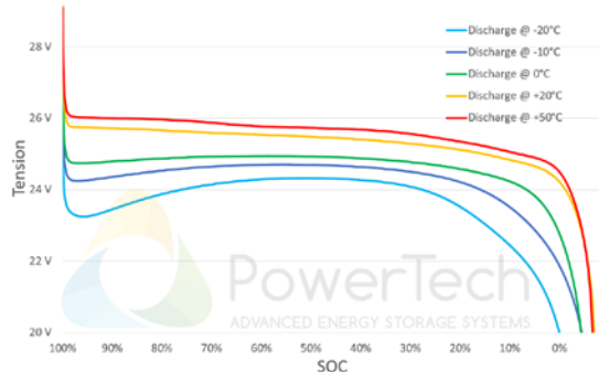
Courbes de décharge (0.5C) à différentes températures
